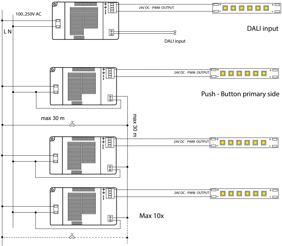
PBOX15D2B PBOX20D2B
